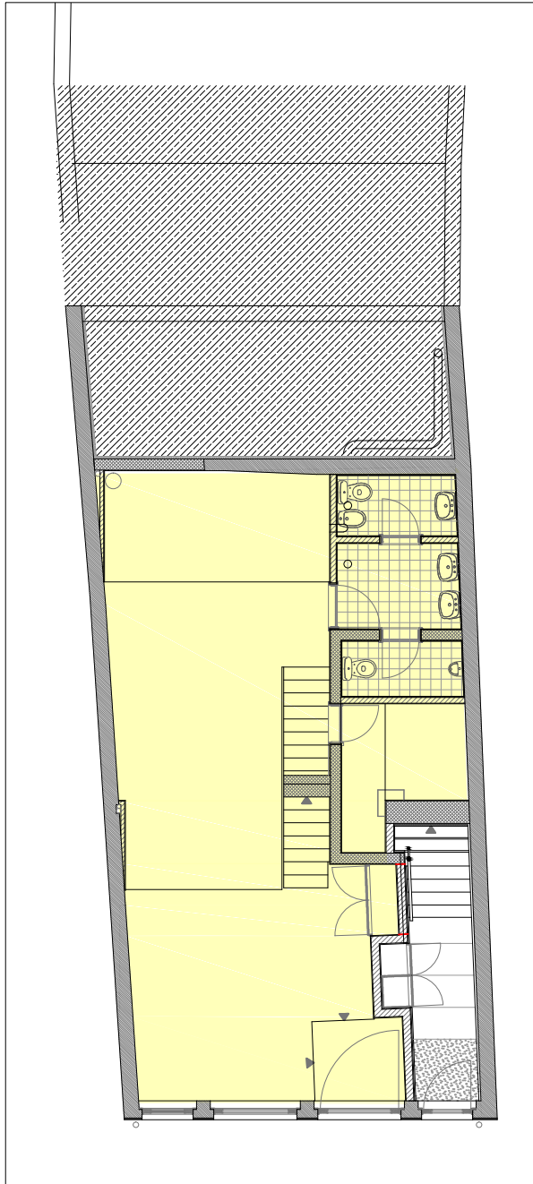
PLANTA (R/CH) - SEM ESCALA
